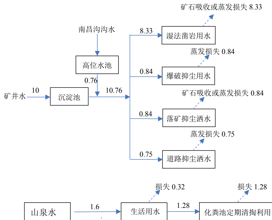
图 1.1 项目水平衡图 （单位：m³/d）
