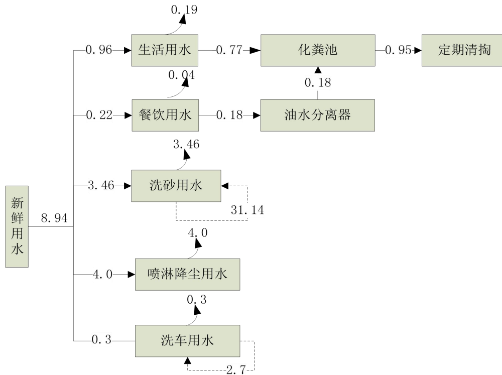
图 1-1 建设项目水平衡图 单位：m³/d
