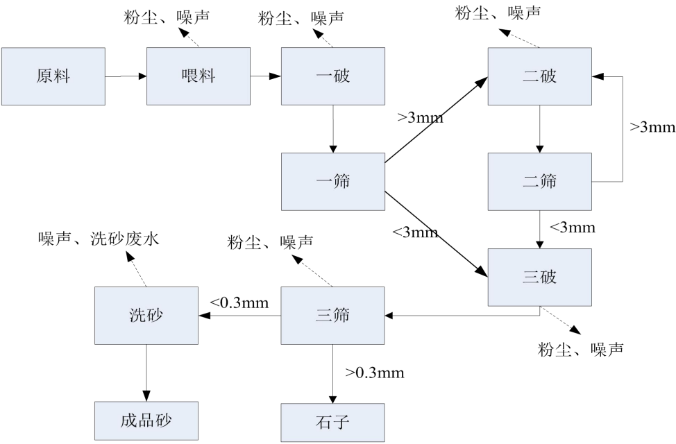
图 5-1 本项目生产工艺流程及产污环节图
