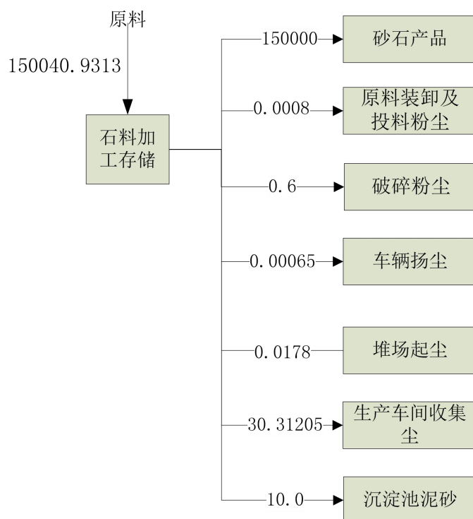
图 5-2 项目物料平衡图
