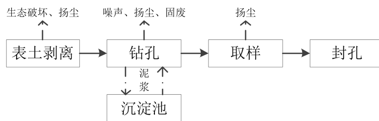
图 5-2 钻探工程工艺流程图
