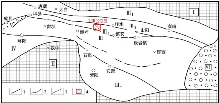
I. 华北地块; II 扬子地块; III 秦岭褶皱系; III 1 . 北秦岭加东褶皱带; III 2 . 礼县—柞水海西褶皱带; III 3 . 南秦岭印支褶皱带; III 4 . 北大巴山加里东褶皱带; IV. 松潘甘孜褶皱系; V. 徽成坳陷; VI. 南阳坳陷; 1. 一级构造单元界线; 2. 二级构造单元界线; 3. 断裂带; 4. 工作区范围
