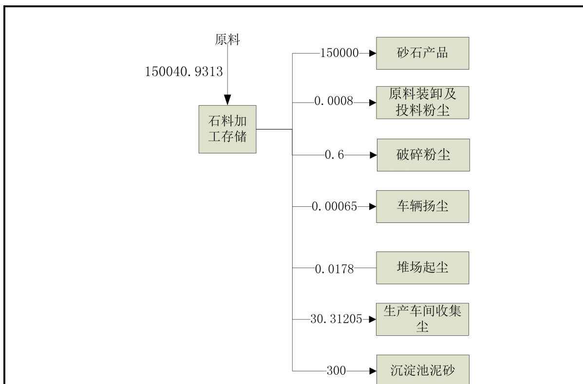
图 5-2 项目物料平衡图
