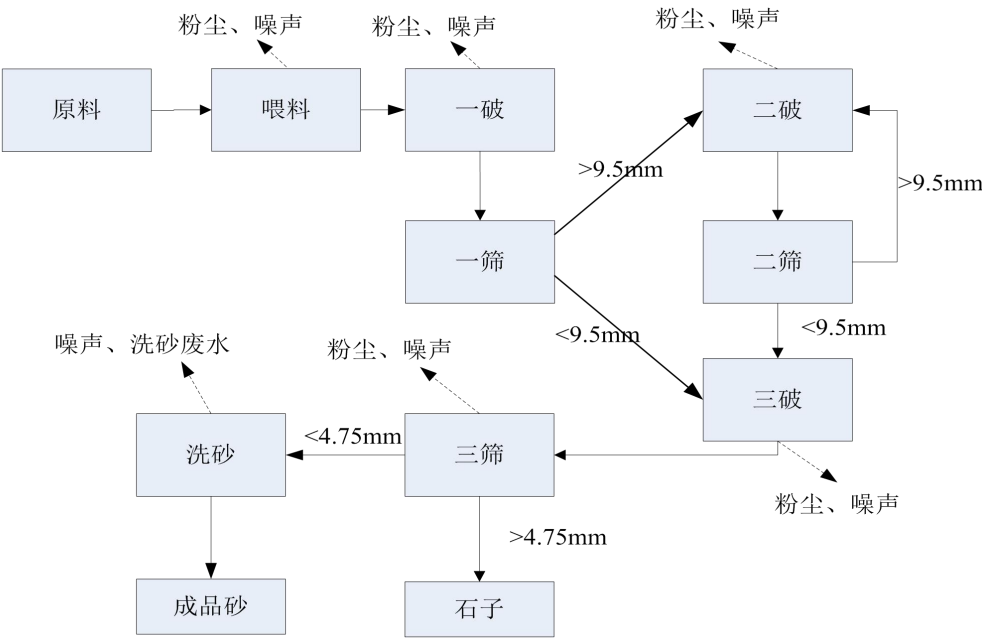
图 5-1 本项目生产工艺流程及产污环节图
