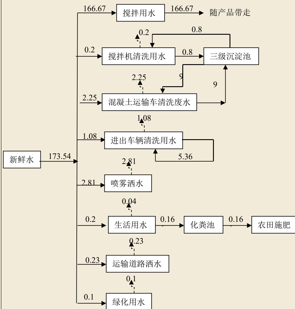
图1 项目区水平衡图 单位: m³/d
