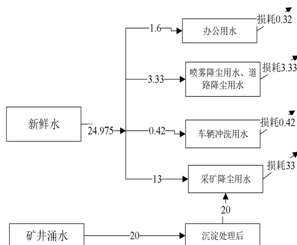
图 2-2 工程生产用水水量平衡图（单位：m 3 /d）
