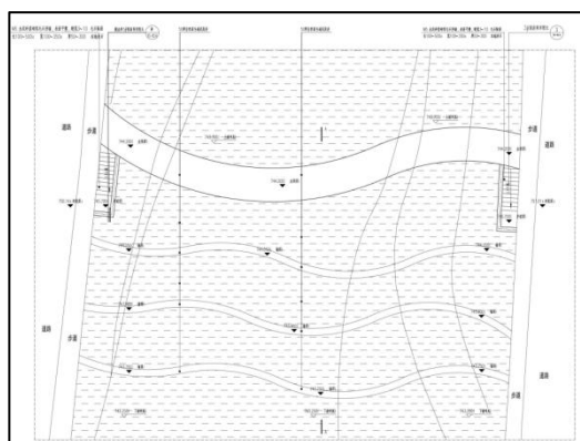
3#固床坝平面设计图
