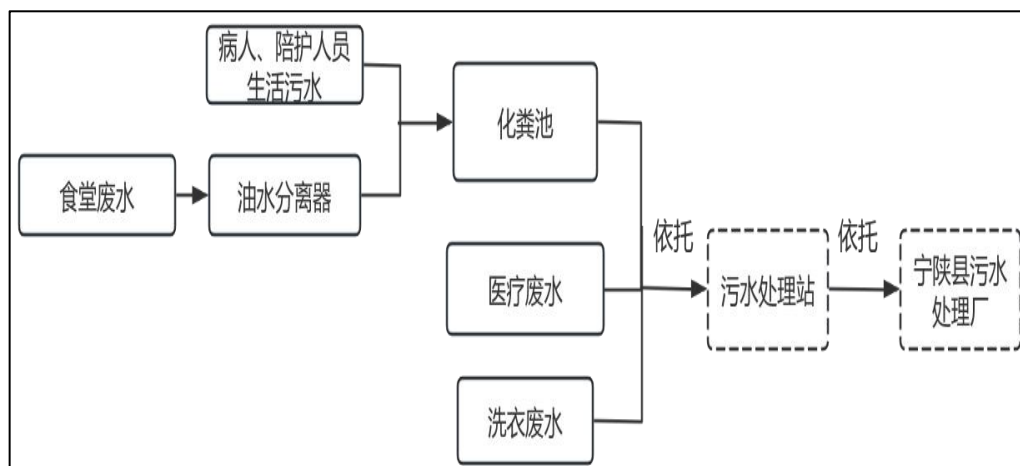
图4.1 本项目废水处理工艺
