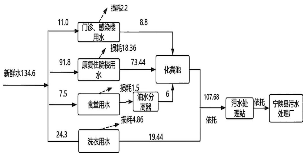
图 2.1 本项目水平衡示意图（单位：m³/d）
