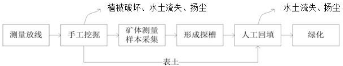
图 2-2 槽探施工流程及产污环节示意图
